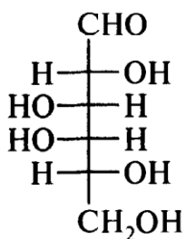
D-галактоза
