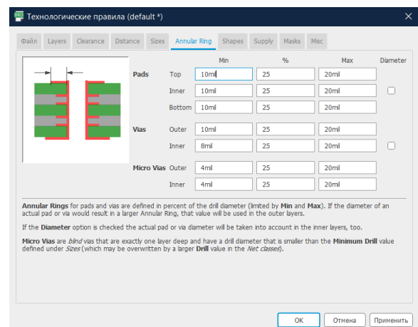
Примеры настроек правил в CAD Eagle
