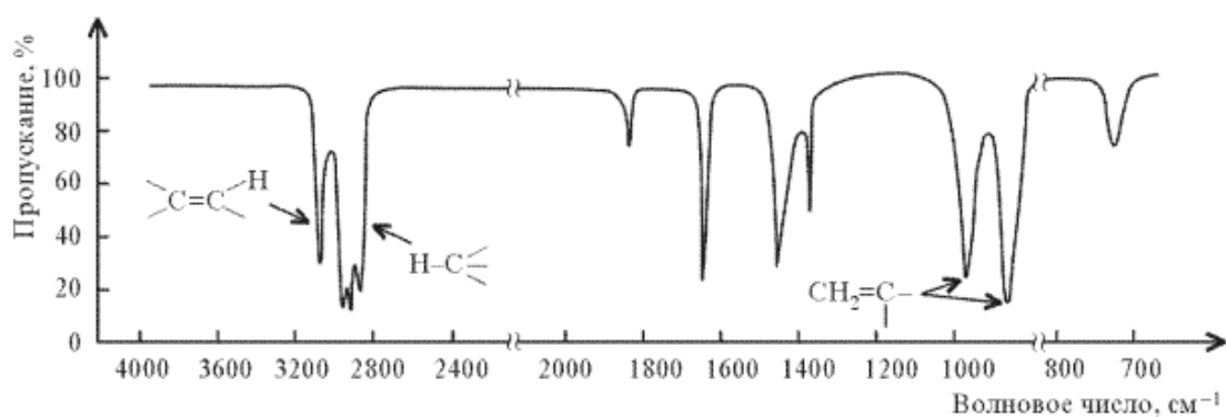
Рис. 2. ИК-спектр гексен-1 \text{CH}_2=\text{CH}(\text{CH}_2)_3\text{CH}_3
