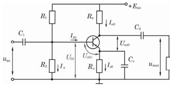
Рис. Схема однокаскадного усилителя ОЭ
