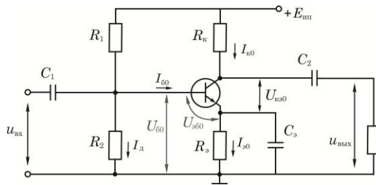
Рис. Схема однокаскадного усилителя ОЭ
