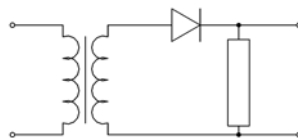
Выпрямитель
