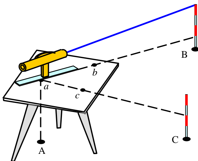
Рис. 10.8 Мензуральная съёмка
