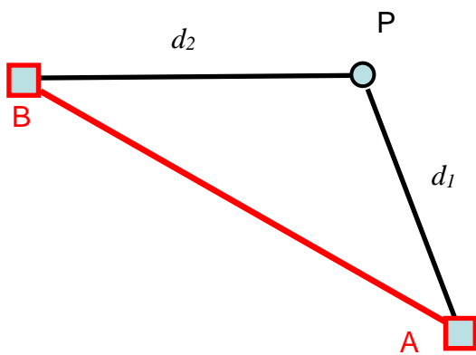
Рис. 10.4 Линейная засечка
