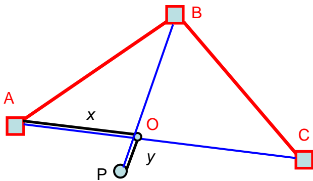
Рис. 10.6 Створная засечка 2
