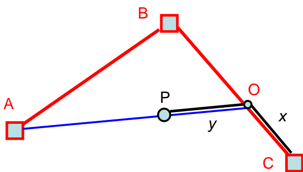
Рис. 10.5 Створная засечка 1
