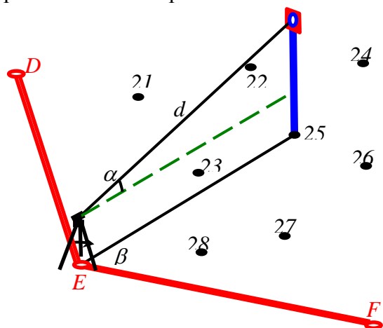
Рис. 10.8 Тахеометрическая
