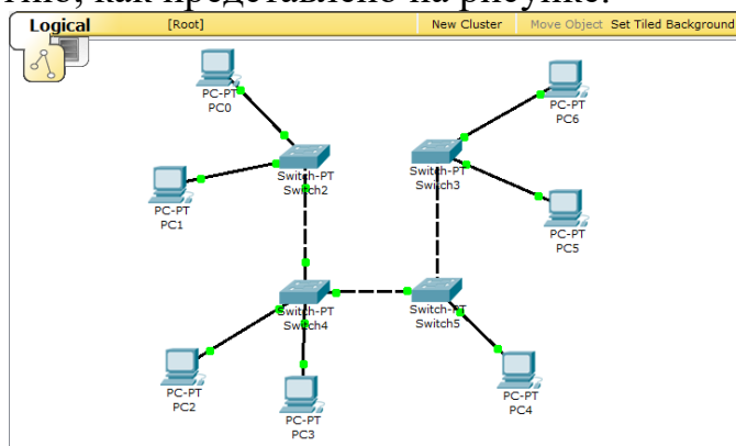
Топология сети для исследования
