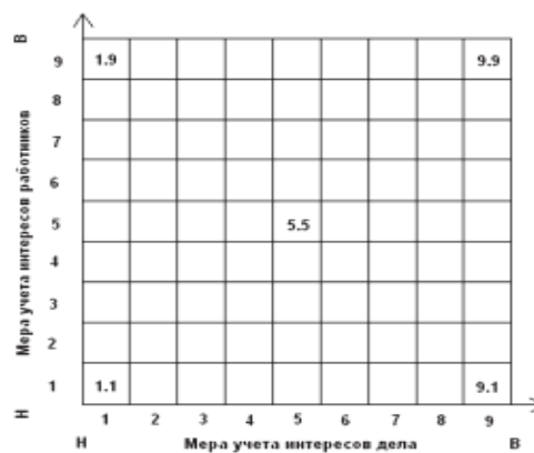
Рис. 2. “Решетка” Блейк-Моутон: Н – низкая; В – высокая
