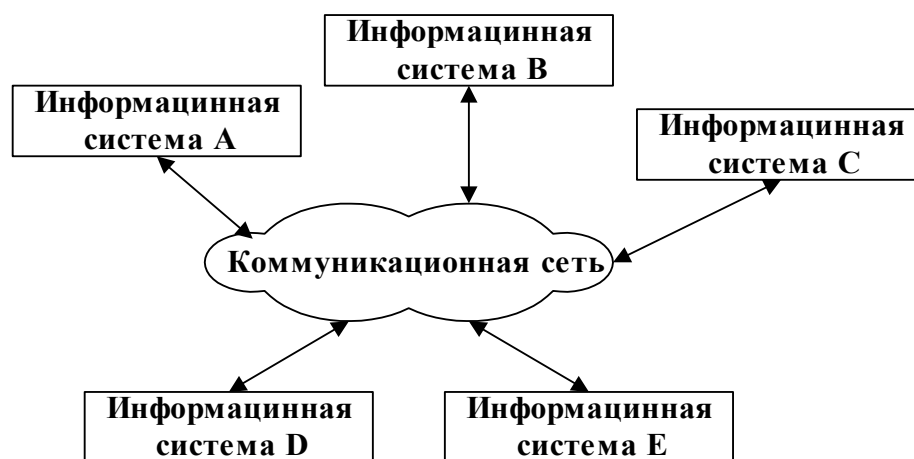
Рис. 1.4 Одноранговая архитектура
