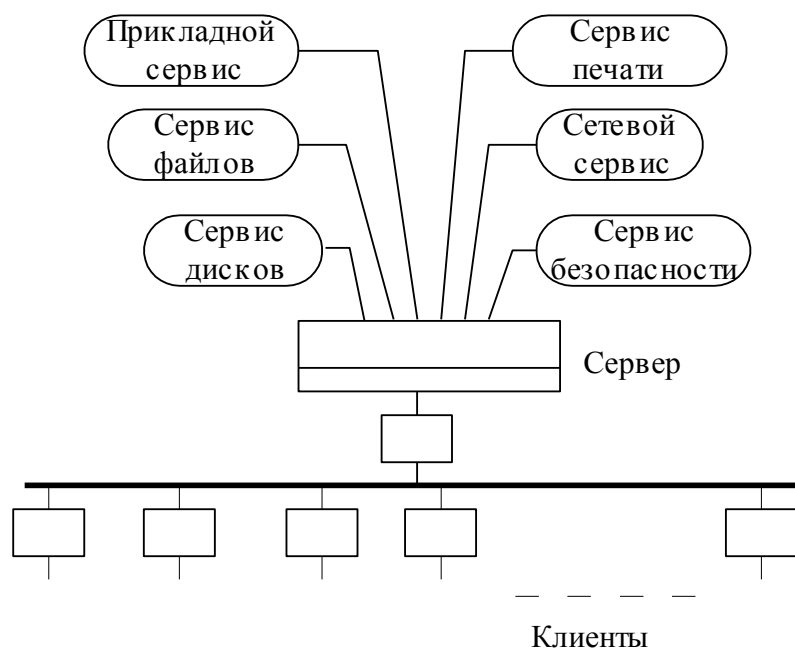
Рис. 1.6 Модель клиент-сервер
